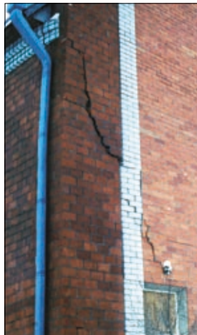
Сквозная трещина на тыльной стороне дома.
