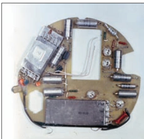
Извлечённая из электросчётчика плата, на которой смонтирован подслушиватель.
