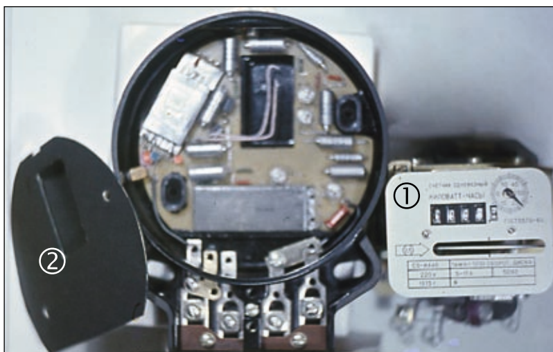
Из корпуса электросчётчика удалён механизм (1) и маскировочная пластина (2), в корпусе виден подслушиватель.
